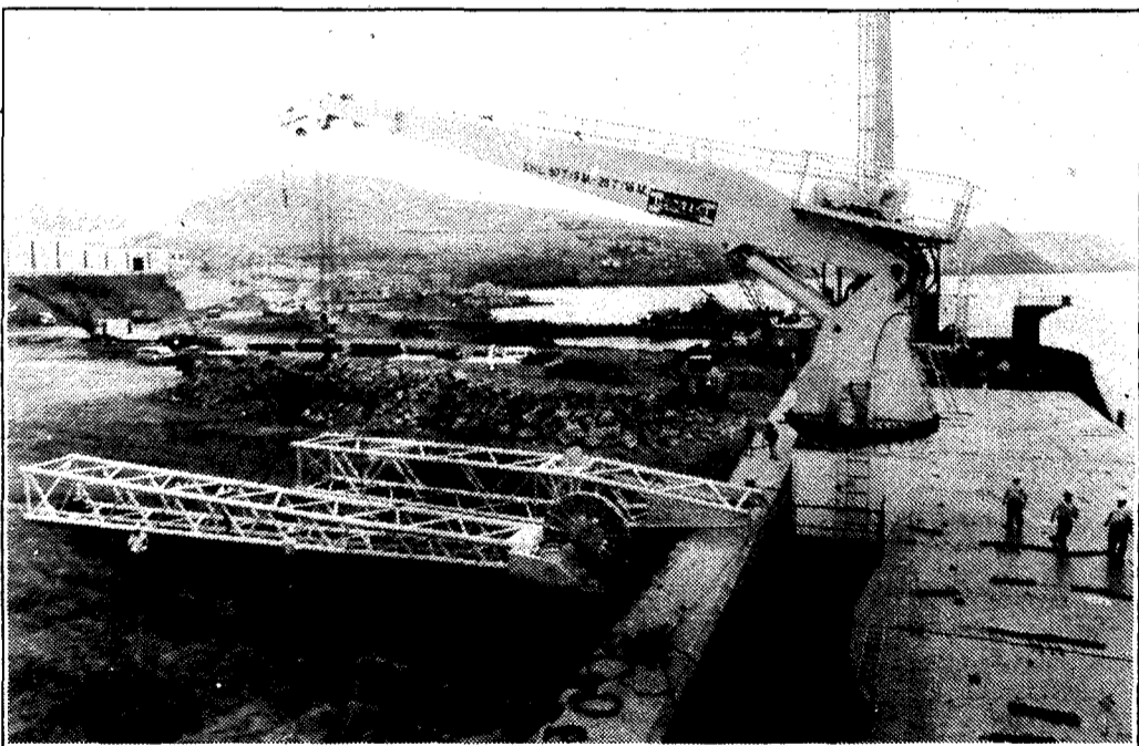
Momento em que se procedia à descarga da grua, em peças separadas.
