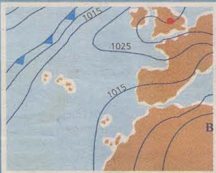
Carta de prognóstico de superfície válida para 15/3/99, às 12 horas locais.
