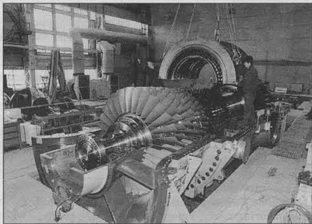
Uma turbina a gás fabricada pela Siemens/LMZ.
