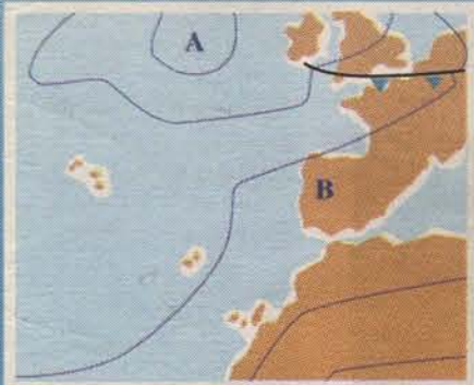
Carta de prognóstico de superfície válida para 21/5/98, às 12 horas locais.
