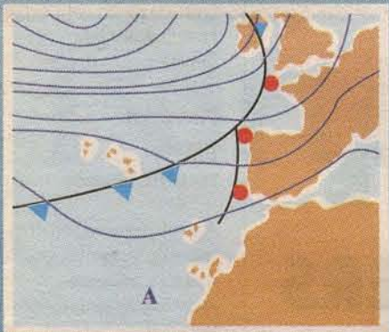
Carta de prognóstico de superfície válida para 29/11/97, às 12 horas locais.
